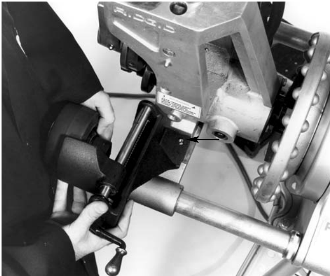
Figure 22 – Alignement des trous de fixation du support sur ceux de l'embase
